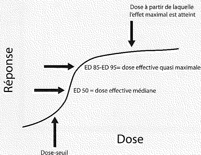
Figure 2: Courbes dose-réponse: sigmoïdale avec un plateau (d'après 7).
